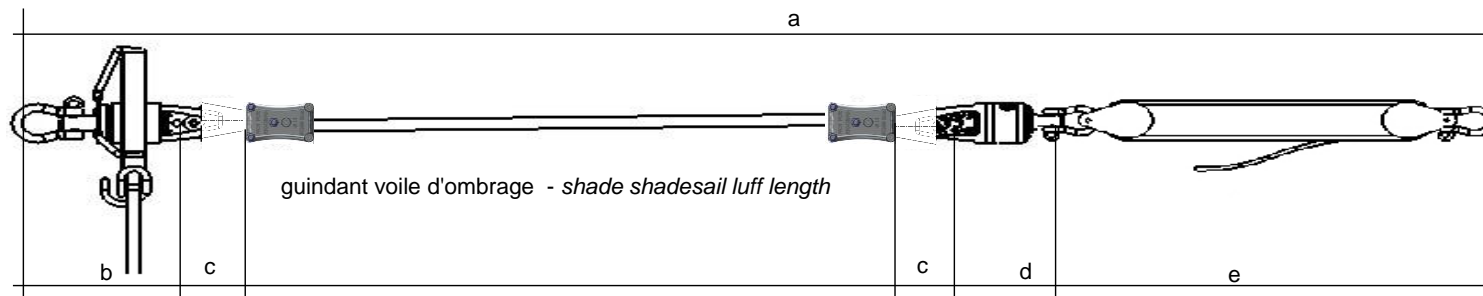
palan pour mise sous tension du câble AT tensioning device for tightening the AT rope
