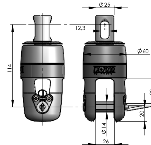
Emerillon / swivel Ref: Poids / Weight : 714g
